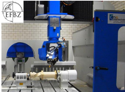
5-Achs-Bearbeitungszentrum
