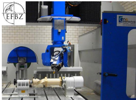
Hauseigenes 5-Achs-Bearbeitungszentrum
