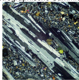
Gesteinsdünnschliff
